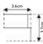
Perfil Vertical
